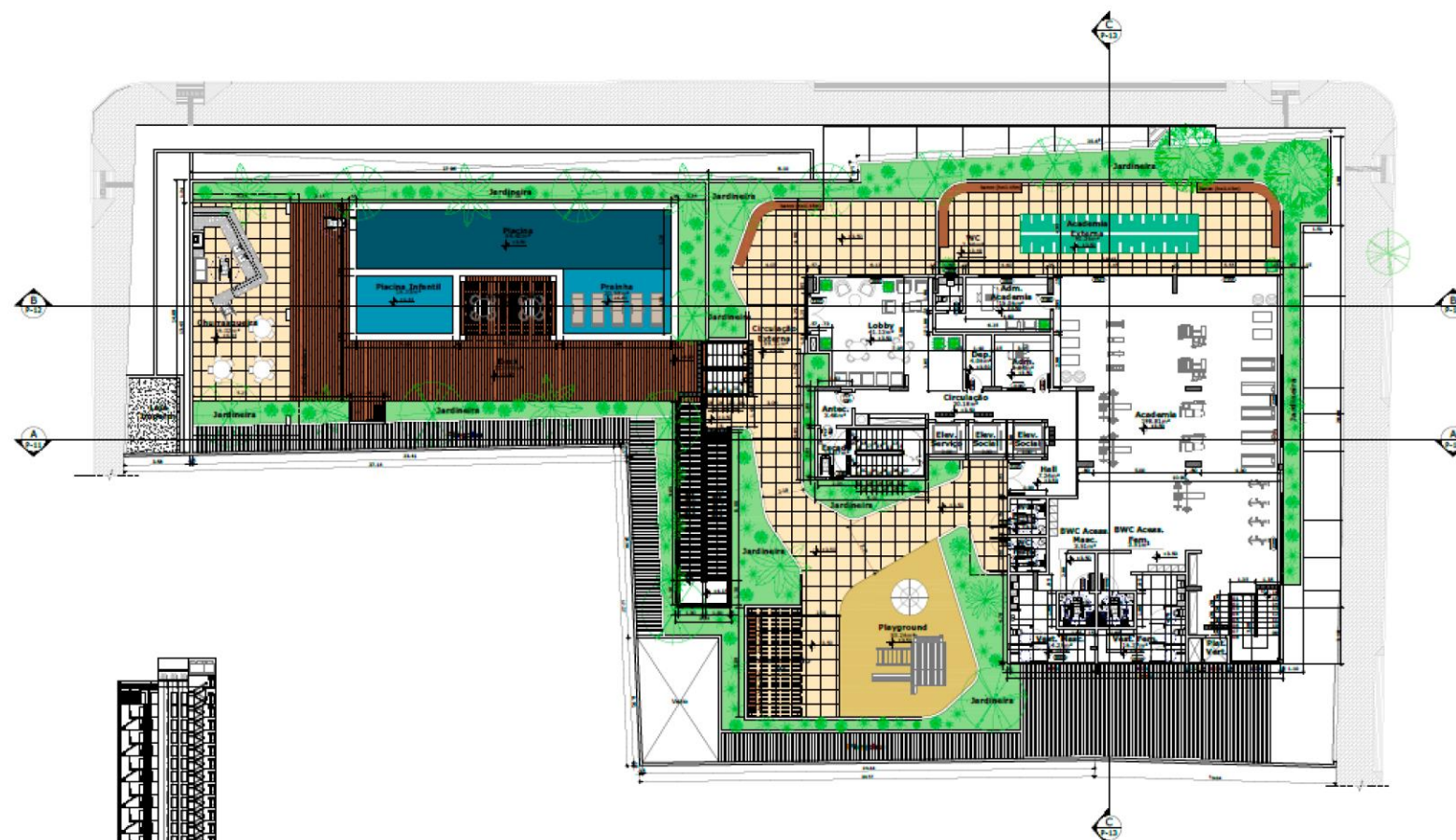
PL BAIXA - 3º PAVTO (LAZER)
