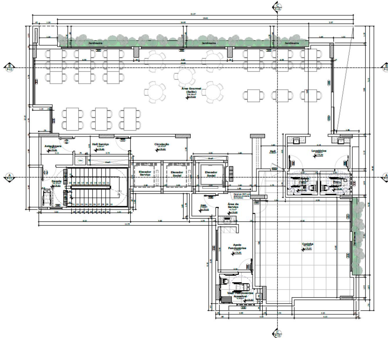
PL BAIXA - 30º PAVTO COBERTURA (ÁREA GOURMET)
