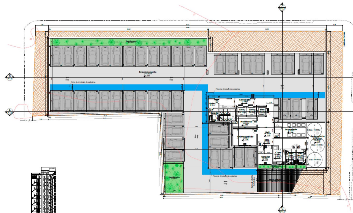
PL BAIXA - 1º PAVTO (SUBSOLO)
