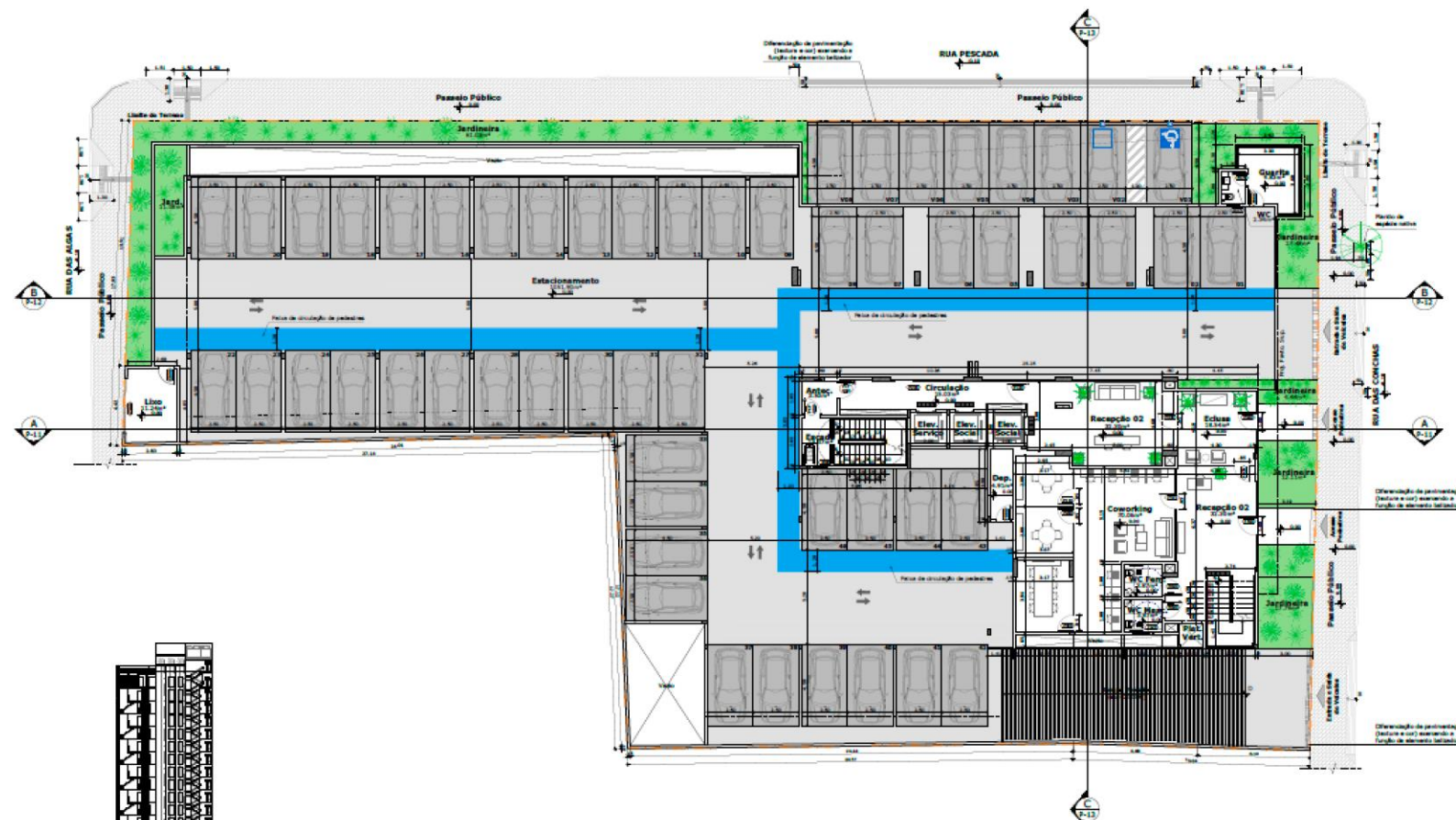
PL BAIXA - 2º PAVTO (TÉRREO)
