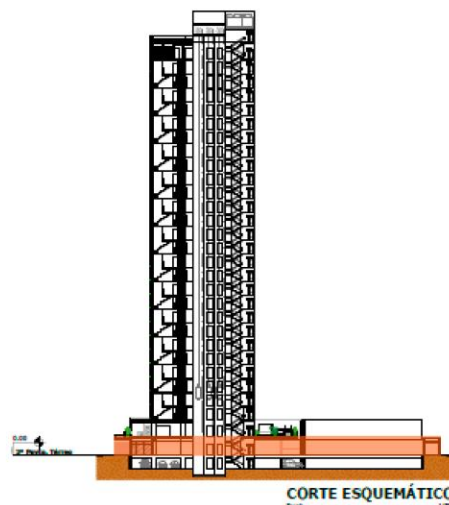
CORTE ESQUEMÁTICO
